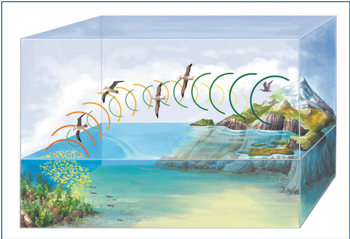
Figure 2. Le paysage olfactif. Les structures bathymétriques tels que les zones de remonté d'eau, les montagnes et les plateaux sous-marins correspondent aux zones productives, où les concentrations de DMS sont les plus élevées, pouvant ainsi servir de point de repère olfactif pour la navigation en mer (De Thivent et Bonadonna, 2003 ©Caroline Picard).
